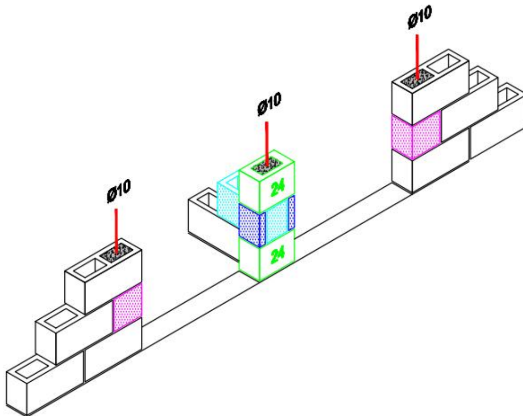
Amarração em Cruz
