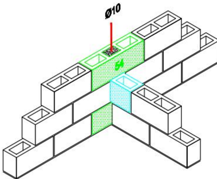
Amarração em T
